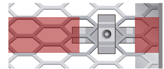
AGARRE Y SOLAPADO (VISTA SUPERIOR)
